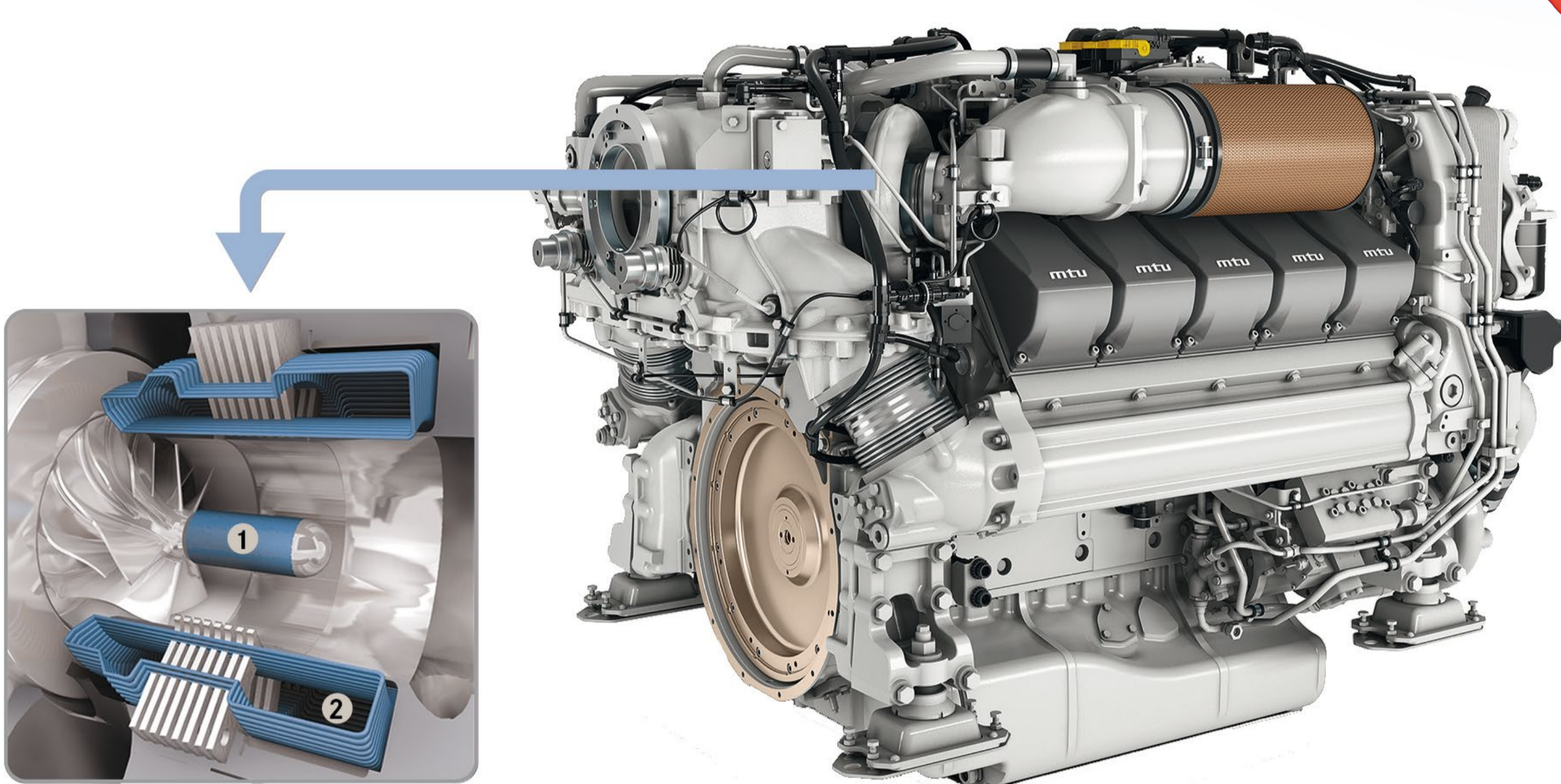
1 Rotor mit Hochleistungsmagnet 2 Statorblech mit Statorwicklung
